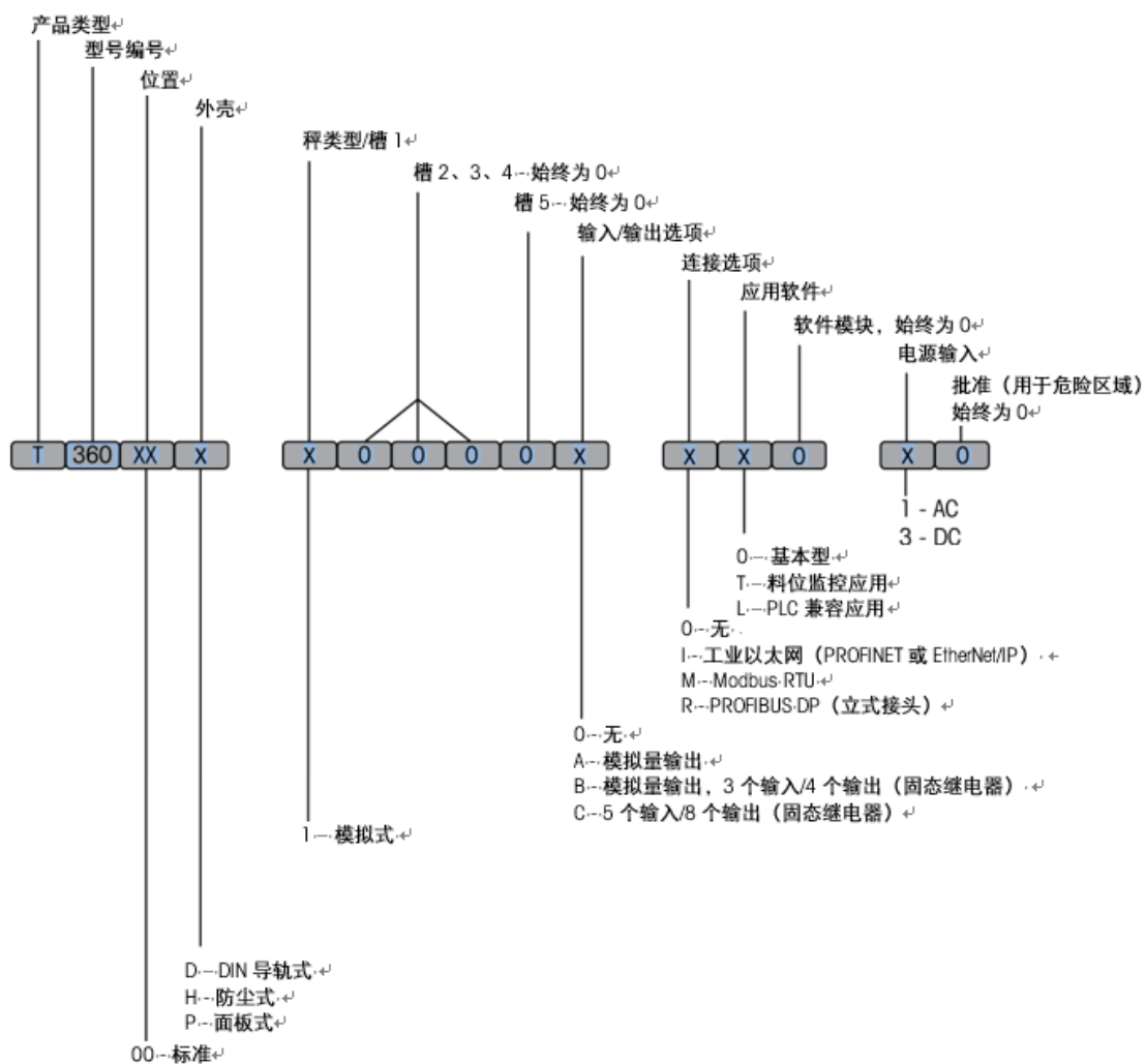
图 1-1: IND360 兼容模式 SCK
